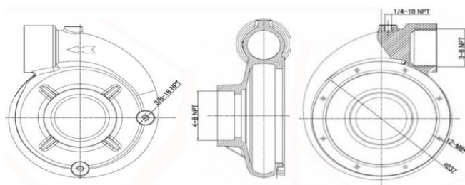
Dimensiones (Tamaño del impulsor 150 mm)
