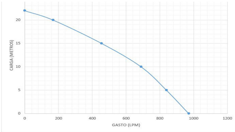
Curva de rendimiento FTB80
