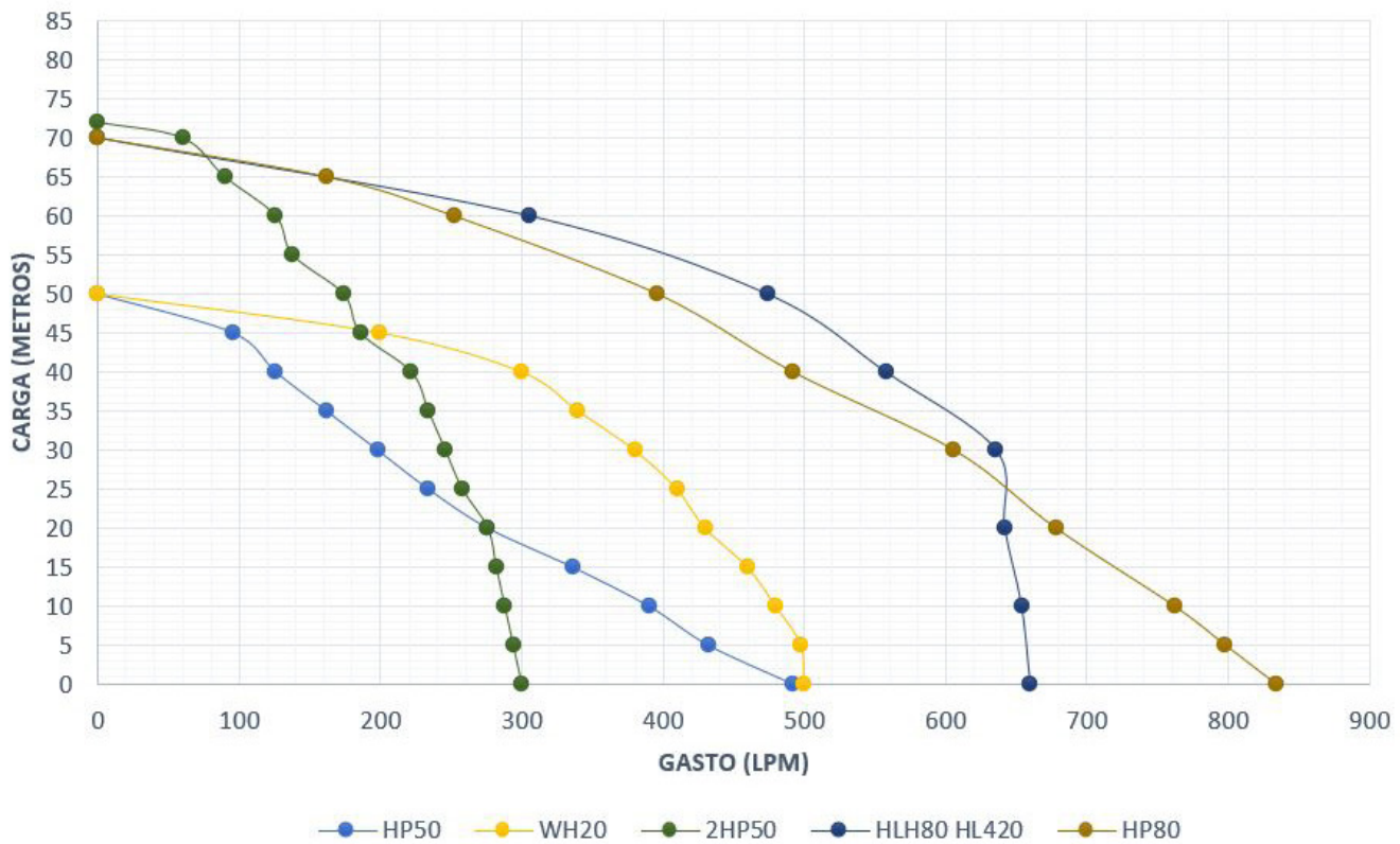
Curvas de rendimiento por familia
