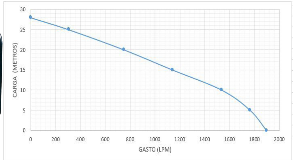
Curva de rendimiento WP150
