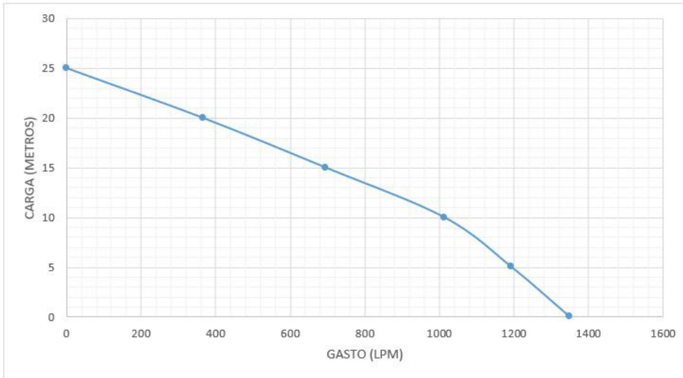
Curva de rendimiento SP80
