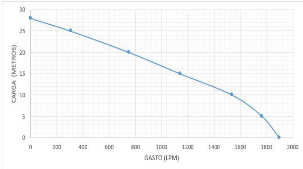
Curva de rendimiento SPI50
