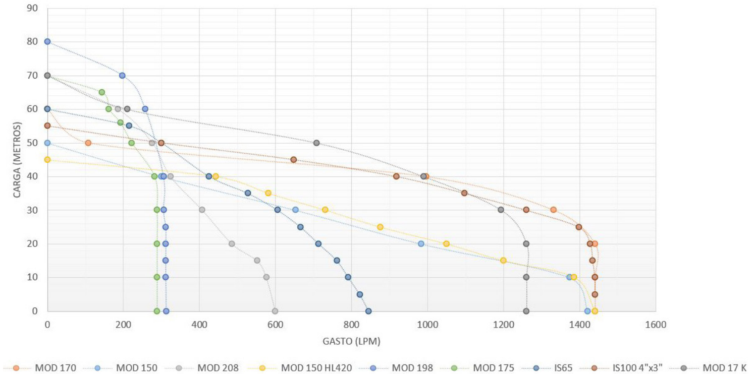
Curvas de rendimiento por familia.
