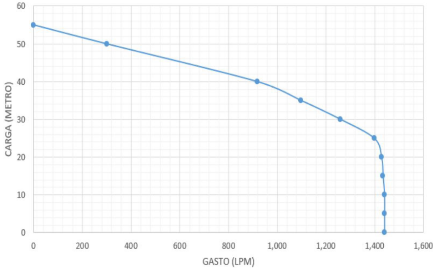
Curva de rendimiento IS 100
