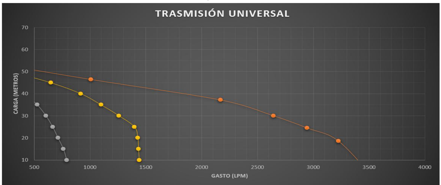
Curvas de rendimiento por familia.
