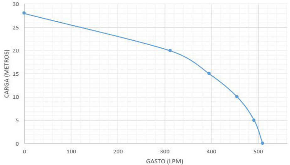
Curva de rendimiento FTB50
