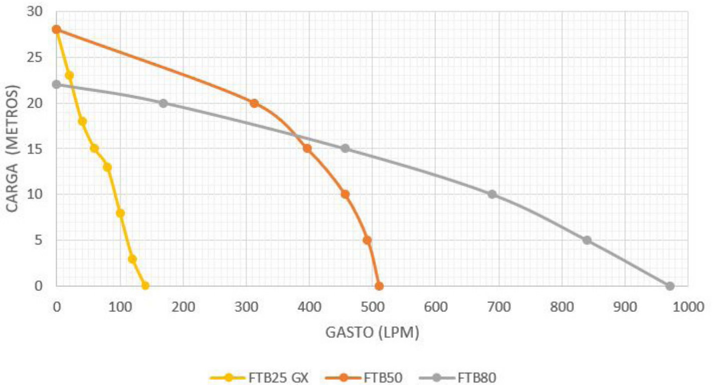
Curvas de rendimiento por familia
