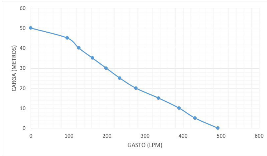
Curva de rendimiento HP50
