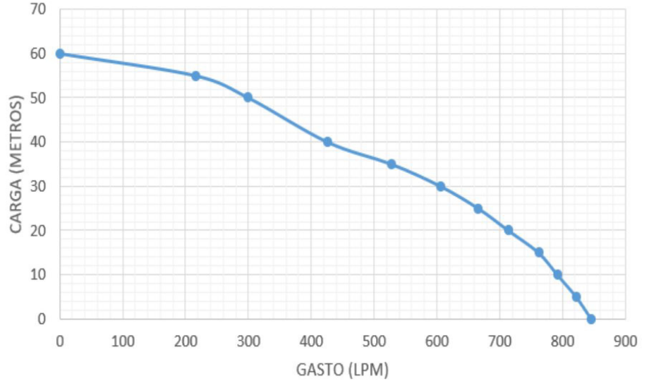
Curva de rendimiento IS 65
