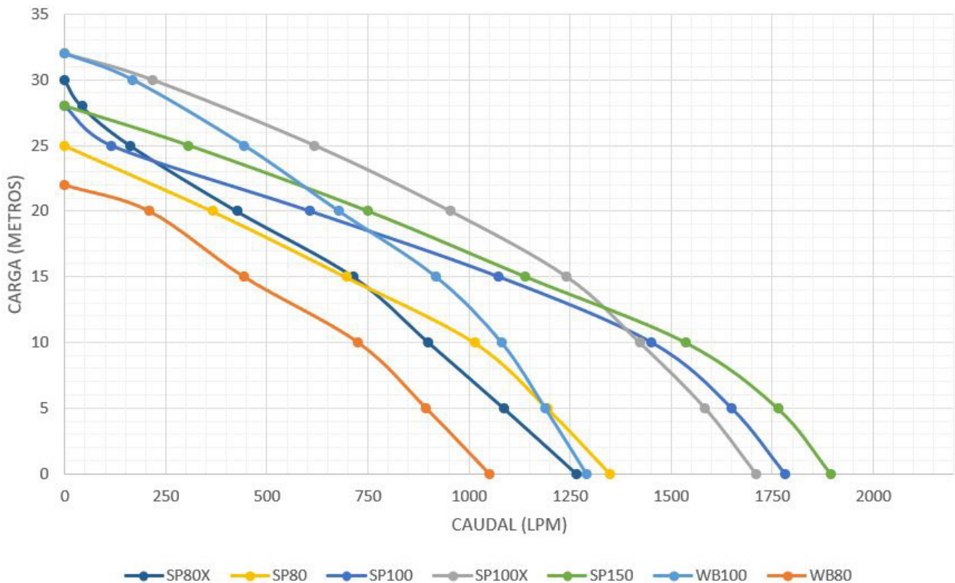
Curvas de rendimiento por familia
