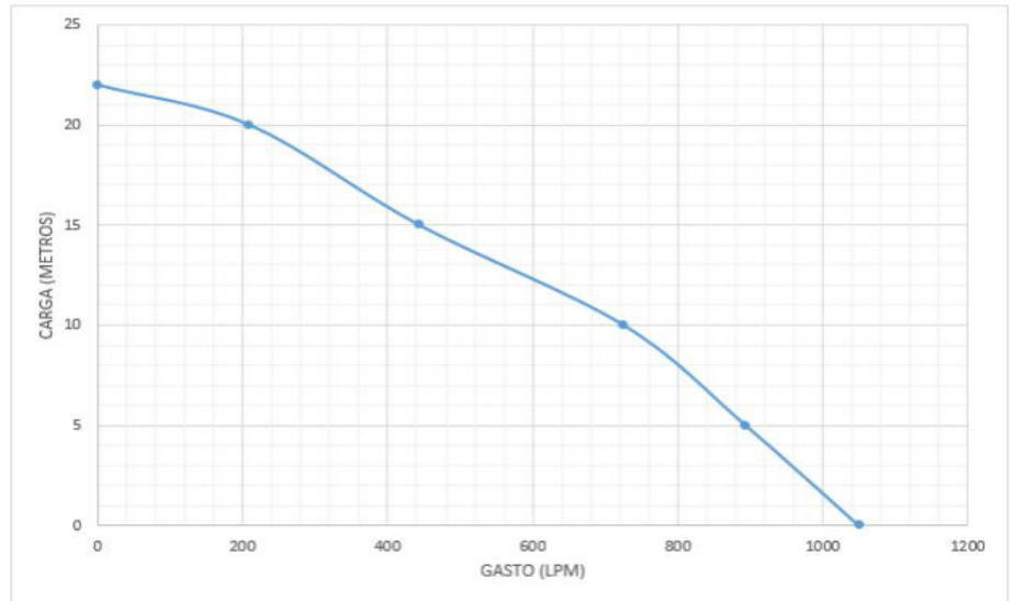
Curva de rendimiento WB80
