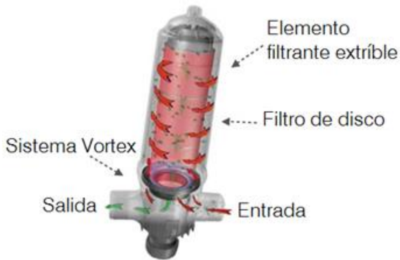
Esquema de funcionamiento modelo F63TD
