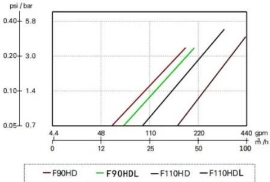
Perdidas de carga para modelos F90HD y F110HDL (120 Mesh)
