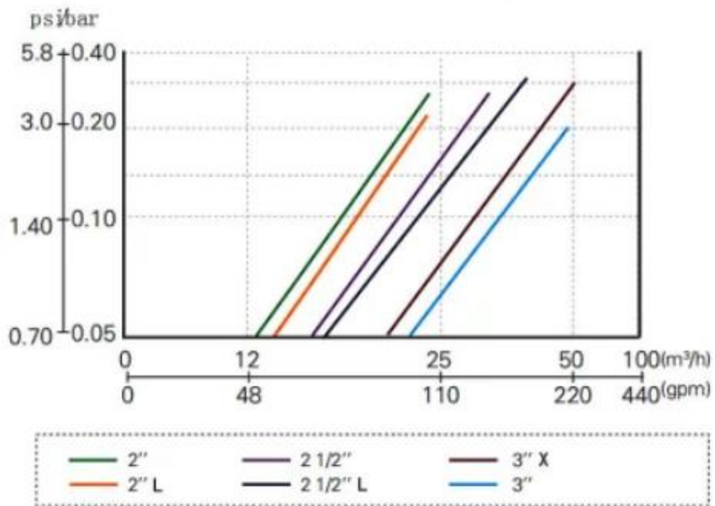
Perdidas de carga para modelo F63TD (120 Mesh)
