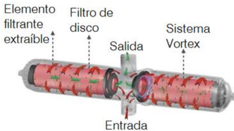
Esquema de funcionamiento modelos F90HD y F110HDL
