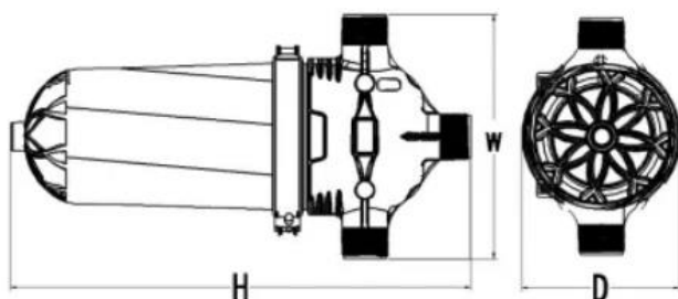
Esquema de dimensiones y conexión de modelo F63TD
