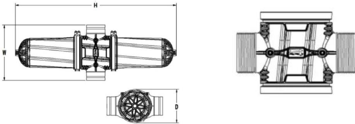
Esquema de dimensiones y conexión de modelos F90HD y F110HDL
